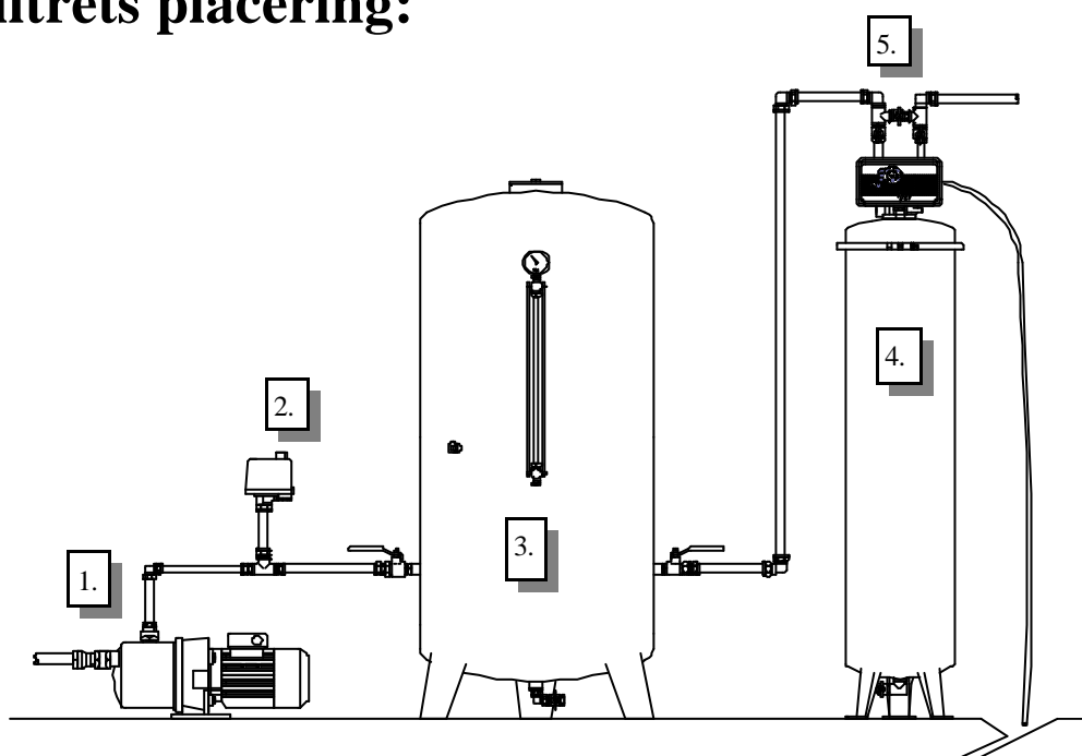
Principskiss
