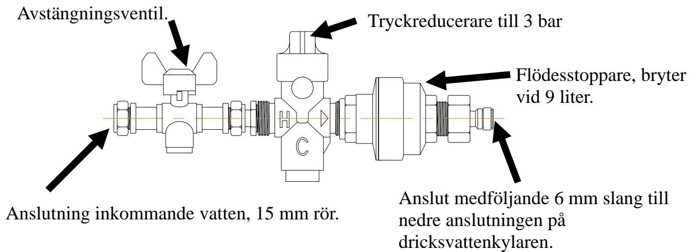
Anslutning vatten från tryck och flödesreguleringspakete
